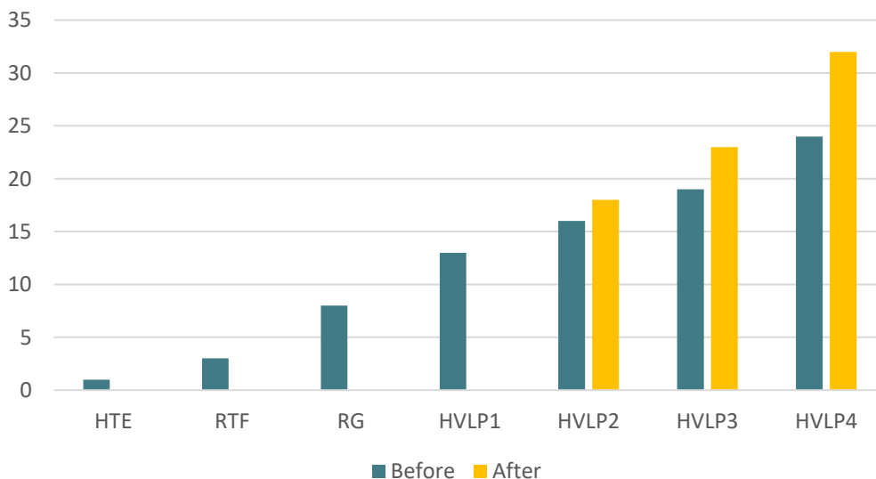
圖五：預期銅箔加工費將持續提升
