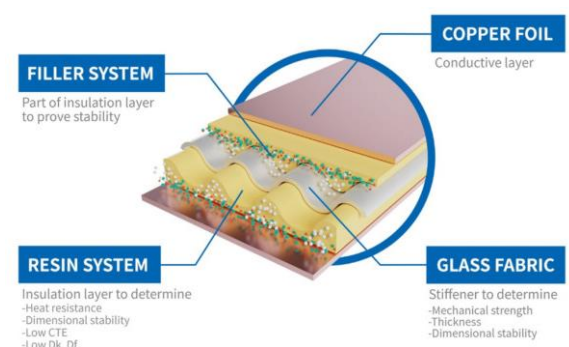
圖二：銅箔基板 CCL
